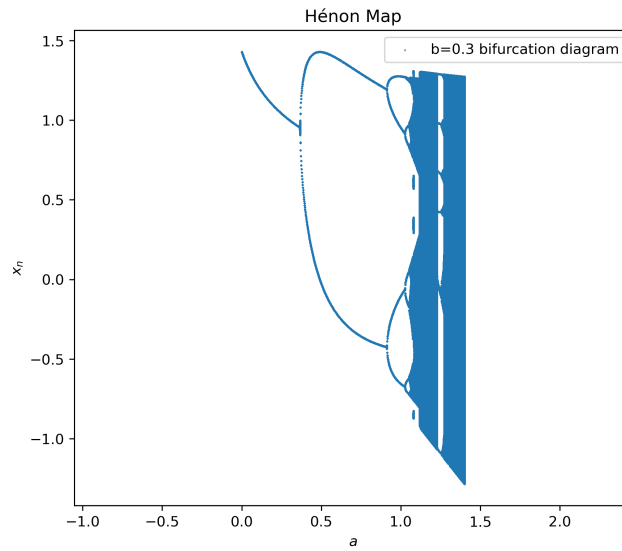
Figure 2: b=0.3 일때 a 값에 따른 x_n 의 갈래치기를 나타낸 그래프이다.
